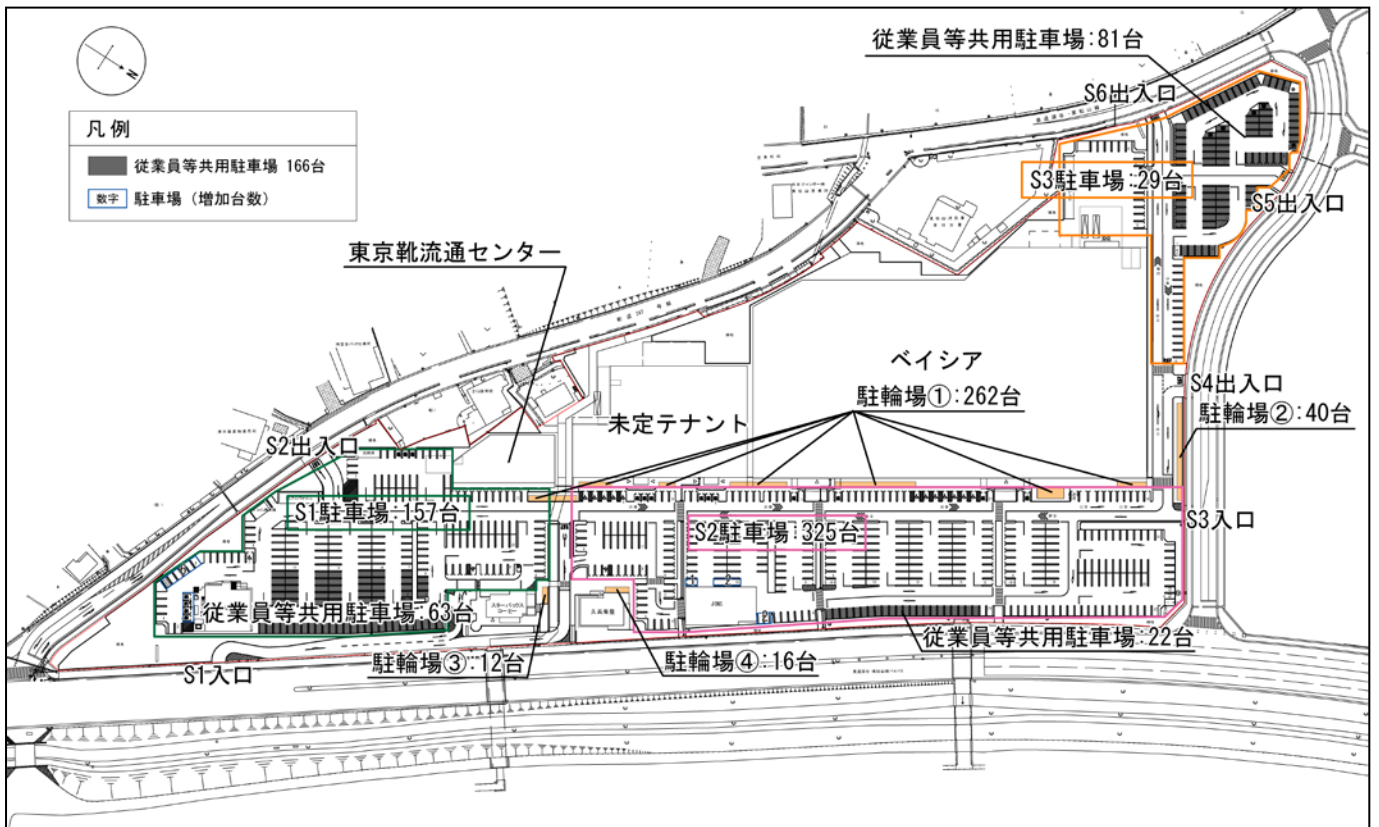
図面 建物配置図及び 1 階平面図（変更後）
